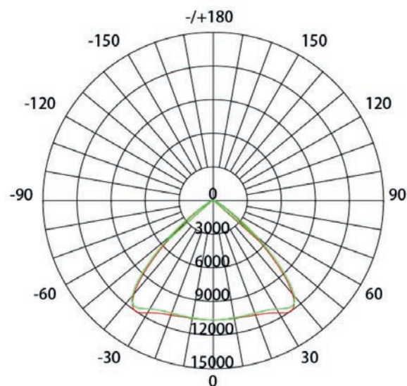
IP69K Highbay Abstrahlcharakteristik
