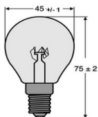
Tropfenform G45 Sockel E14 Dimensionen: 45 * 75 mm Toleranz +/- 2mm
