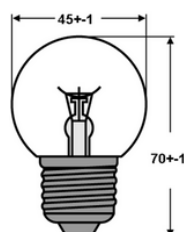
Tropfenform G45 Sockel E27 Dimensionen: 45 * 70 mm Toleranz +/- 1mm
