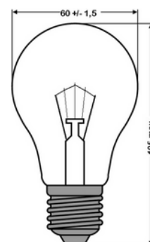
Allgebrauchsform A19 Sockel E27 Dimensionen: 60 * 105 mm Toleranz +/- 1mm
