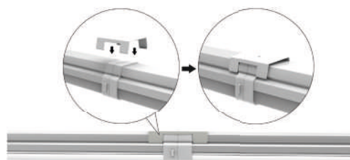
EKSC-BRACKET EKSC-BRACKET-3M
