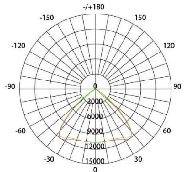
IP69K Highbay Abstrahlcharakteristik
